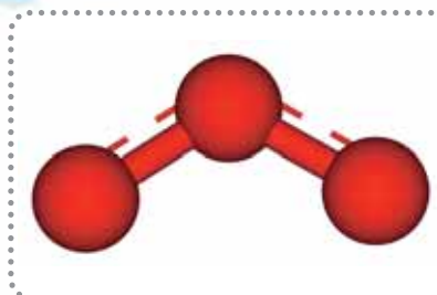
Een ozonmolecule bestaat uit 3 atomen zuurstof. De chemische formule van ozon is O 3 .
